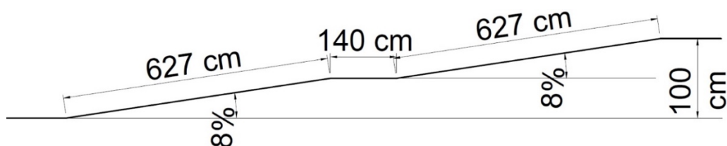
Rysunek 28. Rysunek przykładowych parametrów pochylni o nachyleniu 6% umieszczonych na zewnątrz (bez przekrycia)
